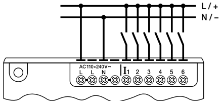
fig. 1. Wiring diagram
