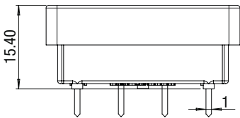
fig. 2. Abmessungen (mm)
