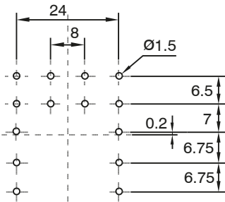
fig. 2. Abmessungen (mm)
