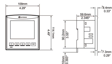
fig. 1. Abmessungen (mm)
