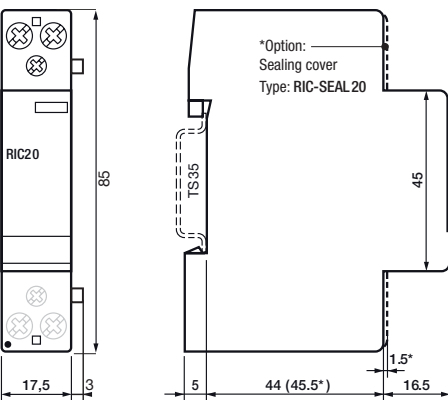
fig. 3. Abmessungen (mm)
