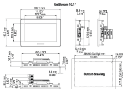
fig. 1. Dimensions (mm)
