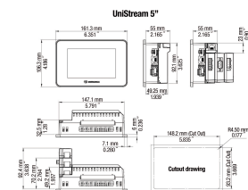
fig. 1. Abmessungen (mm)
