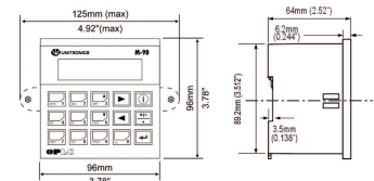
fig. 1. Abmessungen (mm)
