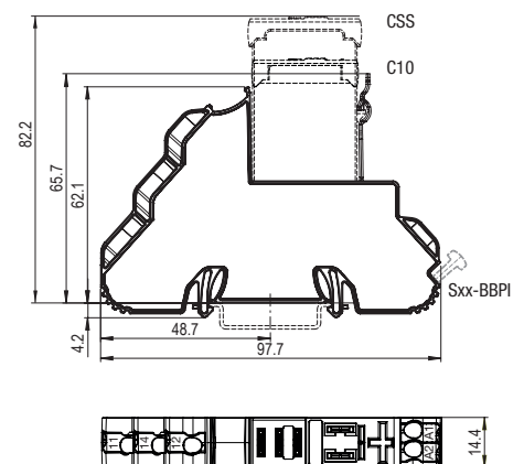
fig. 2. Abmessungen (mm)
