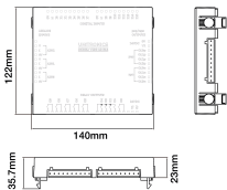
fig. 1. Dimensions (mm)
