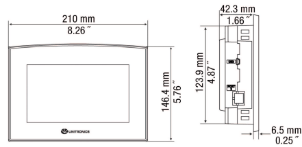
fig. 1. Dimensions (mm)
