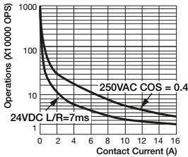
fig. 3. Gleichstrom-Grenzlastkurve
