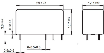
fig. 4. Abmessungen (mm)
