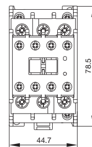
fig. 3. Abmessungen (mm)
