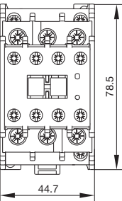
fig. 3. Dimensions (mm)
