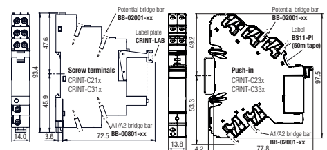
fig. 4. Dimensions (mm)
