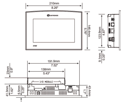
fig. 1. Dimensions (mm)
