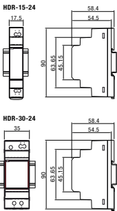
fig. 1. Abmessungen (mm)
