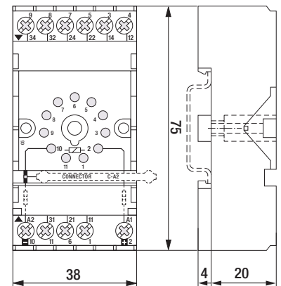
fig. 2. Abmessungen (mm)
