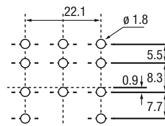
fig. 2. Abmessungen (mm)
