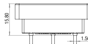
fig. 2. Abmessungen (mm)
