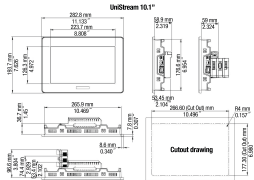
fig. 1. Dimensions (mm)
