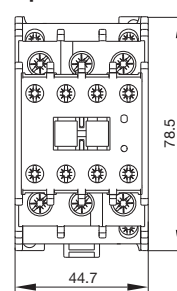
fig. 3. Dimensions (mm)
