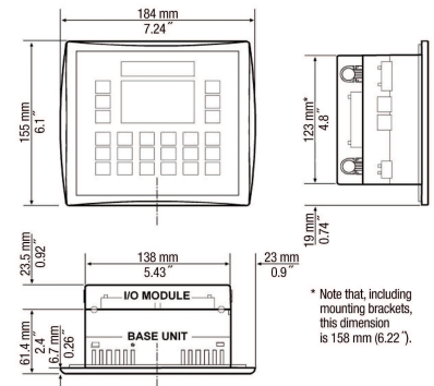
fig. 1. Dimensions (mm)
