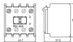
fig. 2. Abmessungen (mm)
