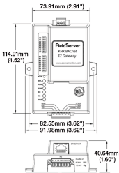
fig. 1. Abmessungen (mm)
