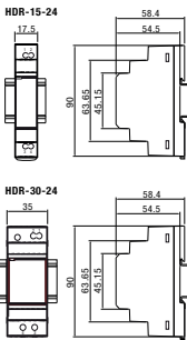
fig. 1. Dimensions (mm)
