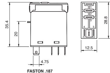
fig. 4. Dimensions (mm)
