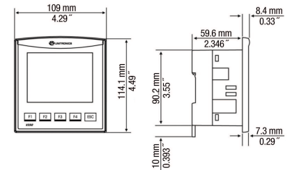
fig. 1. Abmessungen (mm)
