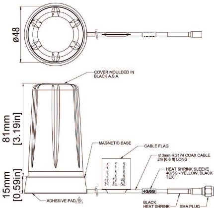
fig. 1. Dimensions (mm)
