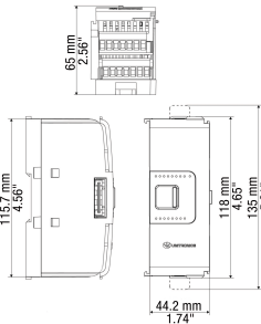
fig. 1. Abmessungen (mm)
