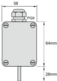
fig. 1. Abmessungen (mm)
