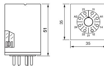
fig. 4. Dimensions (mm)
