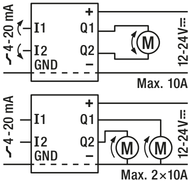
fig. 2. Function diagram
