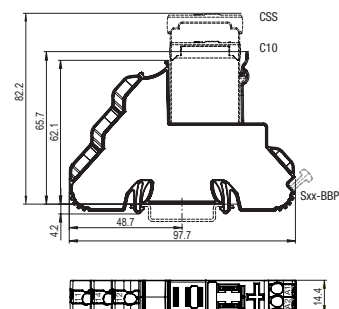
fig. 4. Abmessungen (mm)
