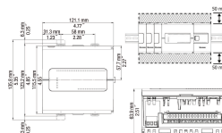
fig. 1. Abmessungen (mm)
