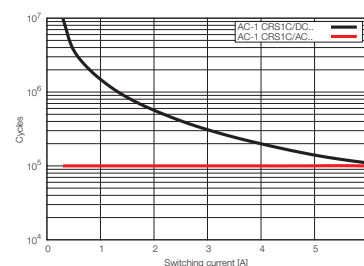
fig. 3. Gleichstrom-Grenzlastkurve
