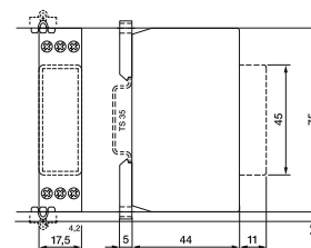
fig. 4. Abmessungen (mm)
