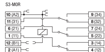
fig. 1. Wiring diagram
