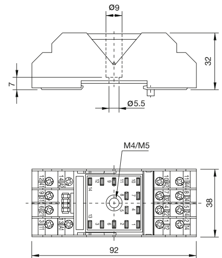
fig. 2. Abmessungen (mm)
