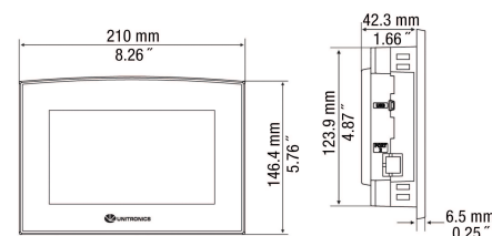
fig. 1. Dimensions (mm)
