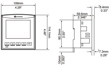
fig. 1. Dimensions (mm)
