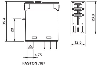
fig. 4. Dimensions (mm)
