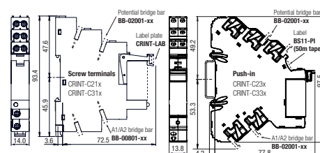
fig. 4. Abmessungen (mm)
