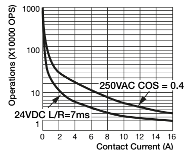
fig. 3. Gleichstrom-Grenzlastkurve
