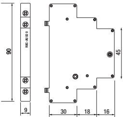
fig. 2. Abmessungen (mm)
