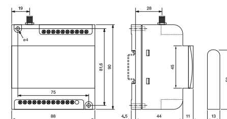
fig. 3. Abmessungen (mm)
