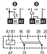
fig. 2. Wechselstrom-Schaltzyklen
