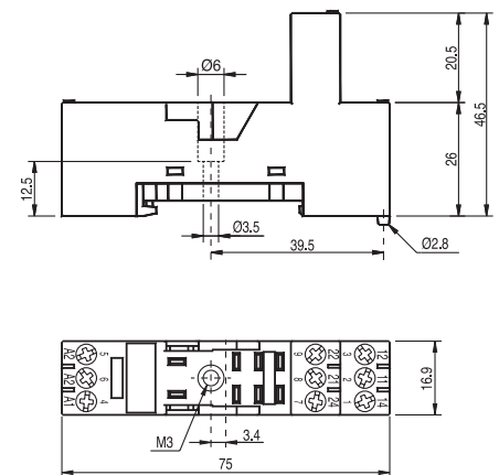
fig. 3. Abmessungen (mm)
