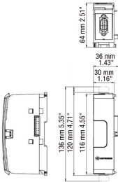
fig. 1. Abmessungen (mm)
