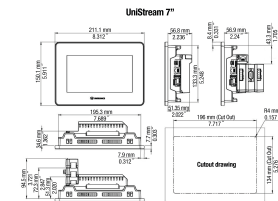
fig. 1. Abmessungen (mm)
