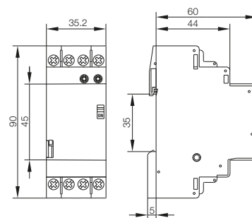
fig. 3. Abmessungen (mm)
