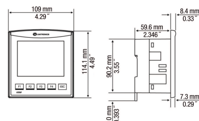
fig. 1. Abmessungen (mm)
