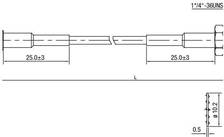
fig. 2. Abmessungen (mm)
