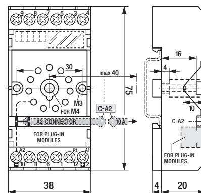
fig. 2. Abmessungen (mm)
