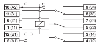
fig. 1. Verdrahtungsdiagramm
